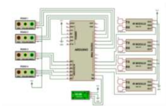
Fig.1. Circuit diagram.
